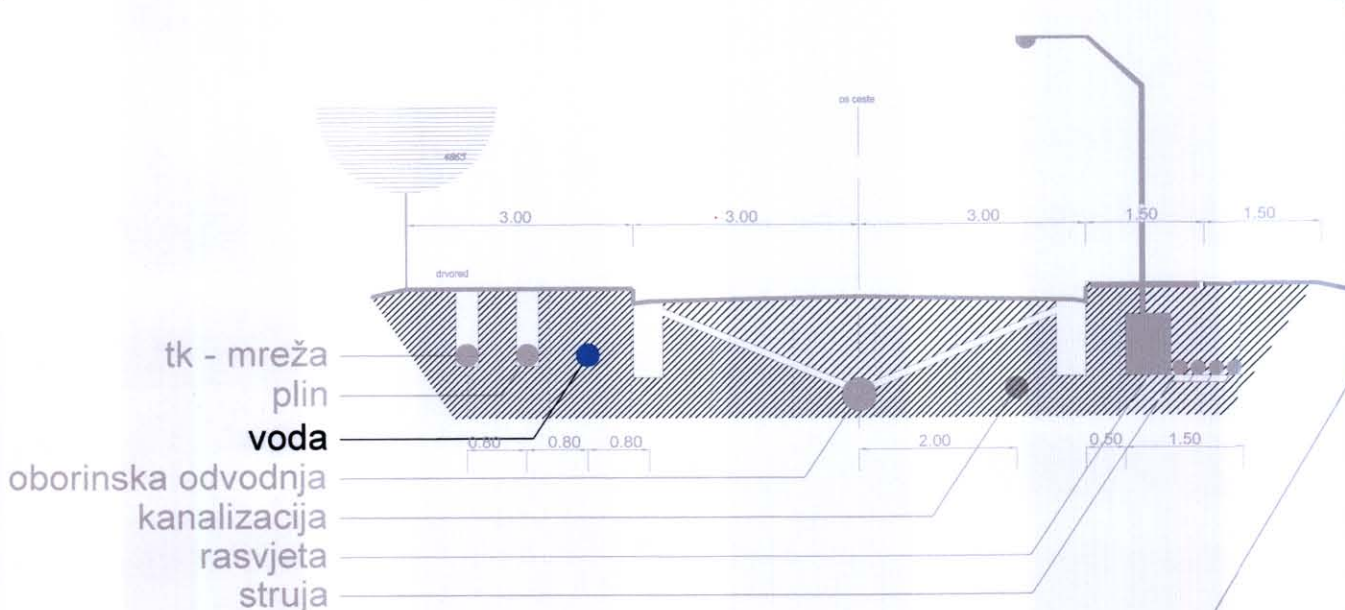
TIPIČAN RASPORED INSTALACIJA U GLAVNIM MJESNIM ULICAMA POPREČNI PRESJEK
